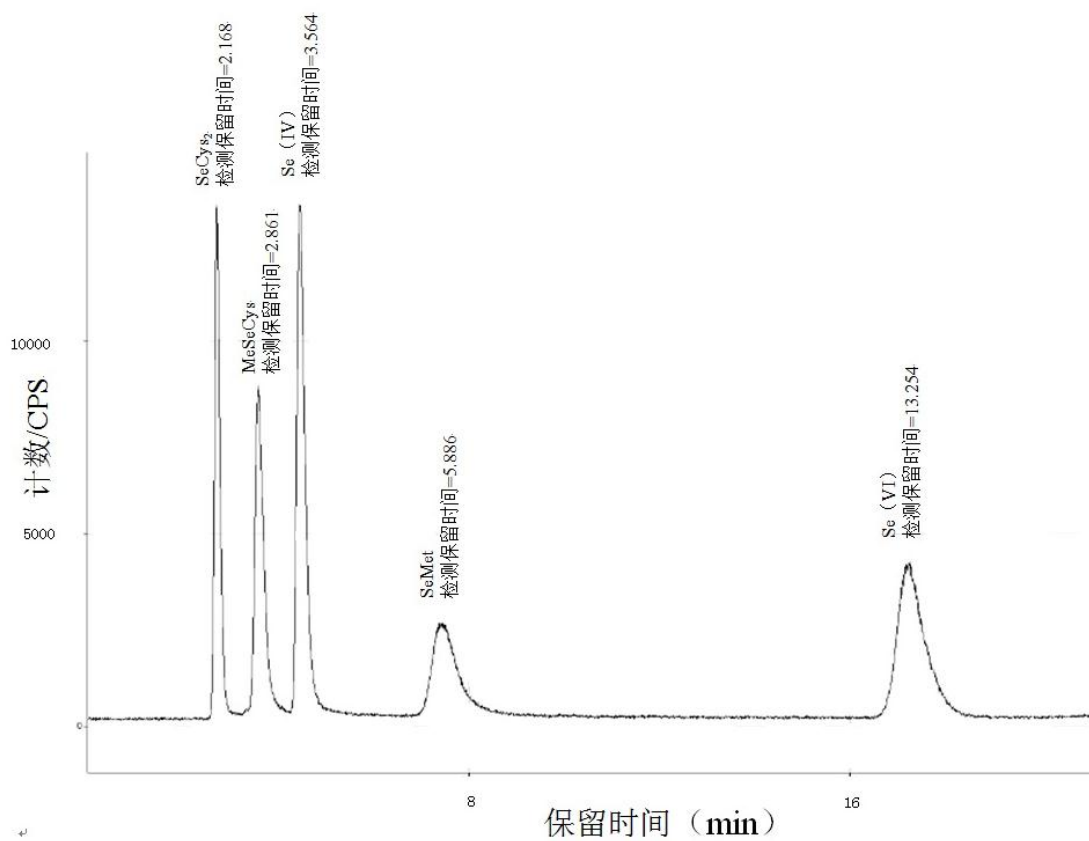
图A.1 5种硒形态标准溶液色谱图
